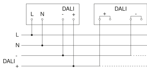
Schema elettrico collegamento in rete di DALI-2 APC & DALI-2 IPD
